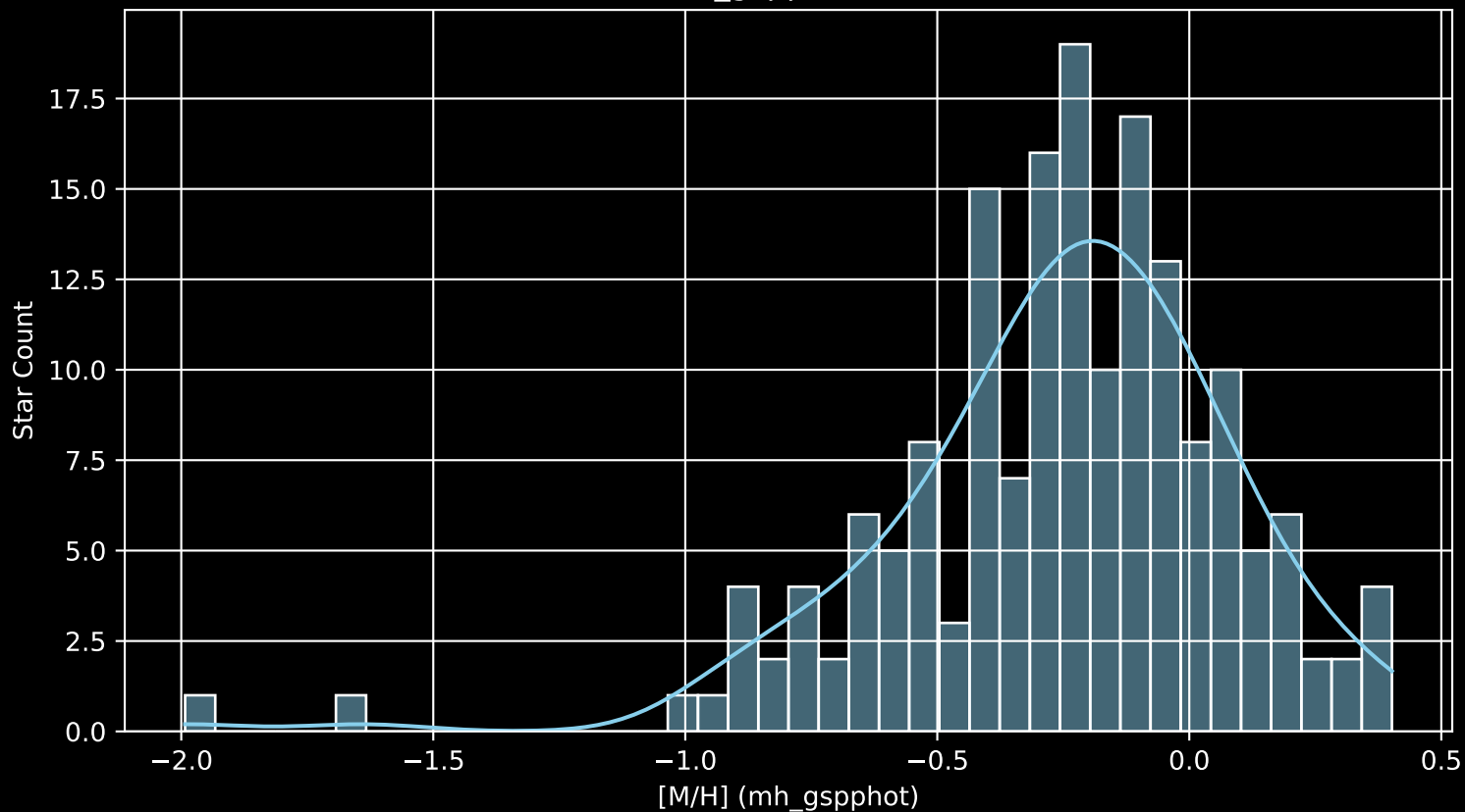
APOGEE DR17 Field: [200+34 MGA [M/H] (mh_gspphot) (n= 172)
